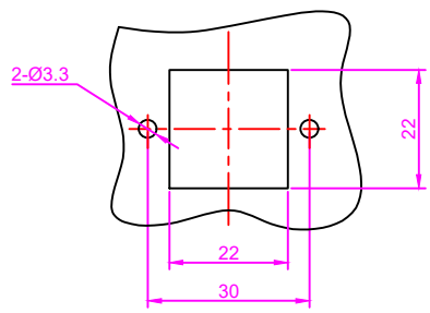
面板开孔图 Panel cut
